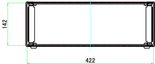
B-B ( 1 : 6 )
