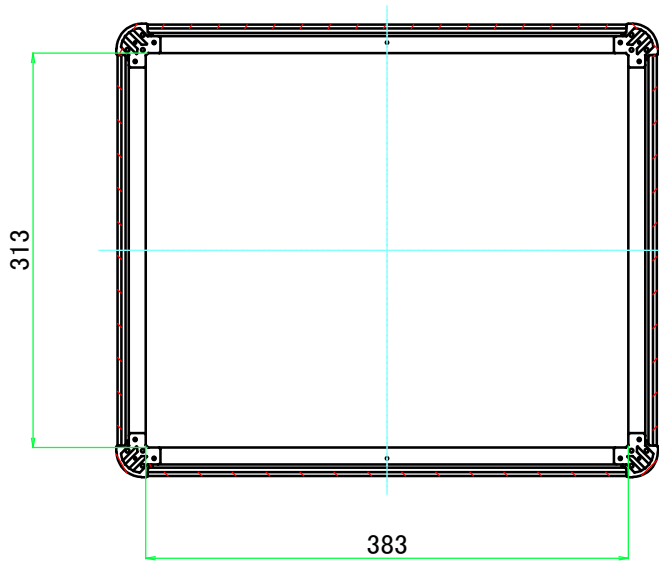
C-C ( 1 : 6 )
