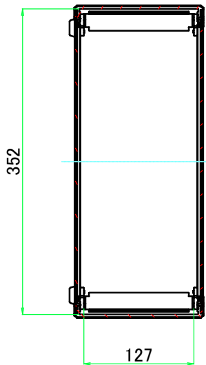
A-A ( 1 : 6 )
